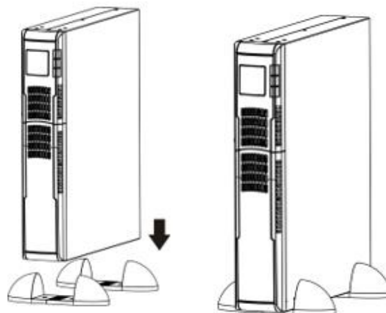
Шаг 2: Установить ИБП на подставки
